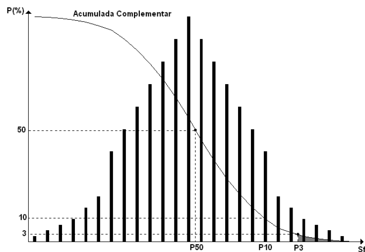
Figura 2 – Distribuição Acumulada Complementar da Sensação de Cintilação
